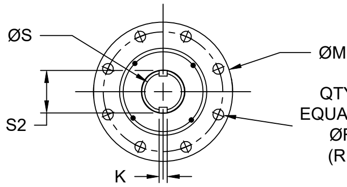
TOP FLANGE
