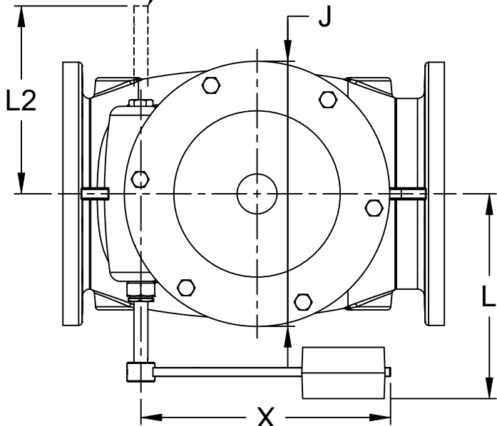
VIEW A-A
